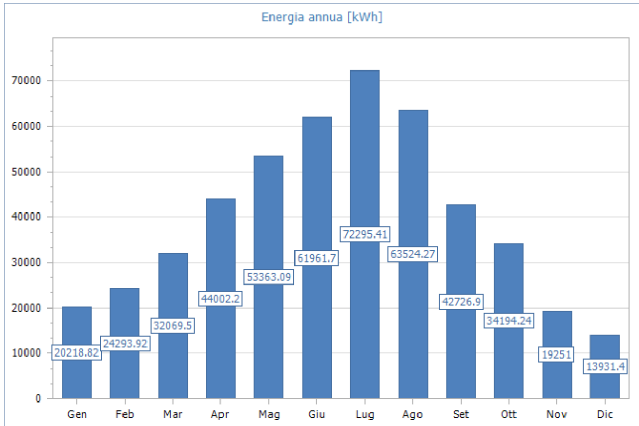
Figura 6 Energia mensile prodotta dall'impianto
